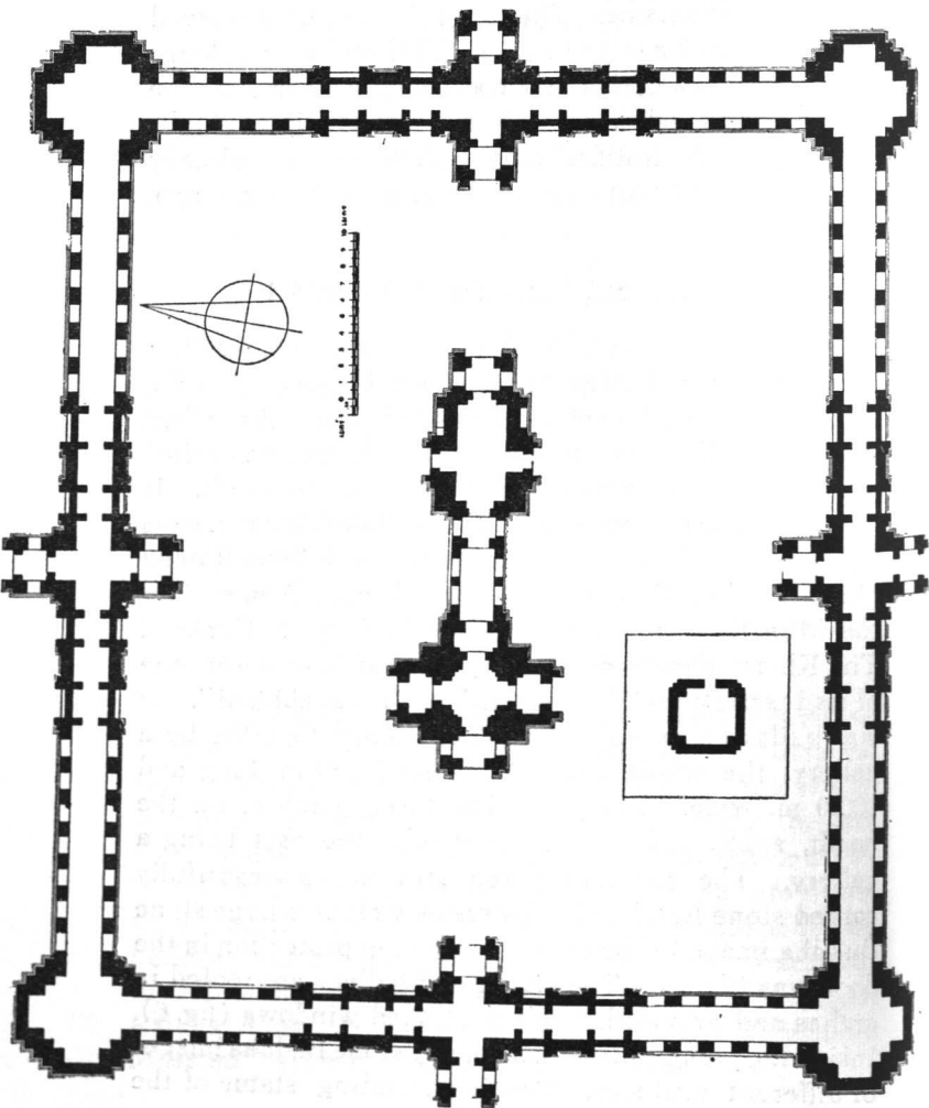
วัดพนมวัน PLAN OF WAT PHANOM WAN จังหวัดนครราชสีมา (KORAT) PROVINCE OF NAKHON RATCHASIMA (KORAT)
